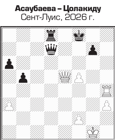
Ход белых
