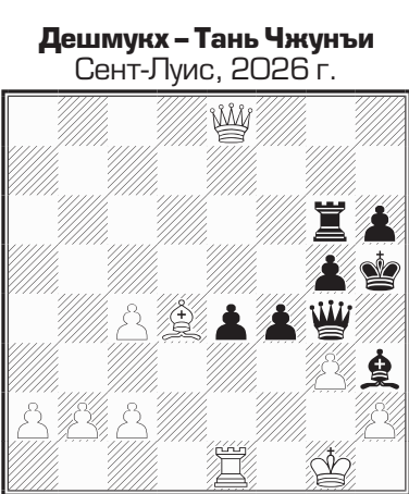
Ход черных
